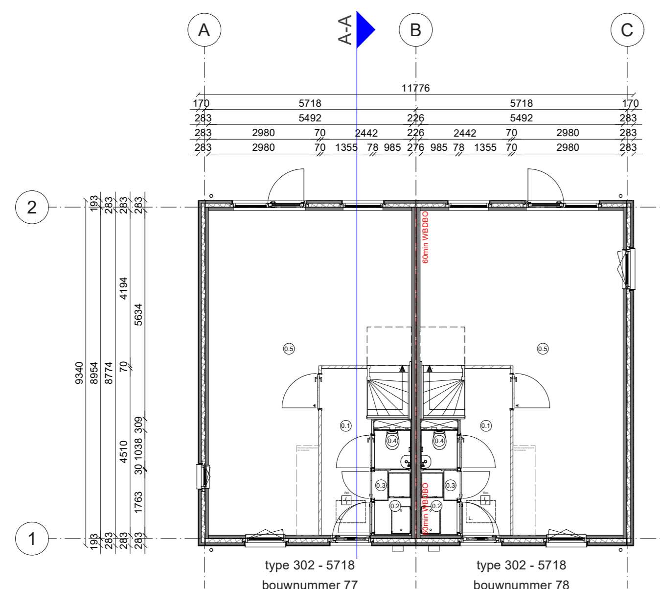
Begane grond
