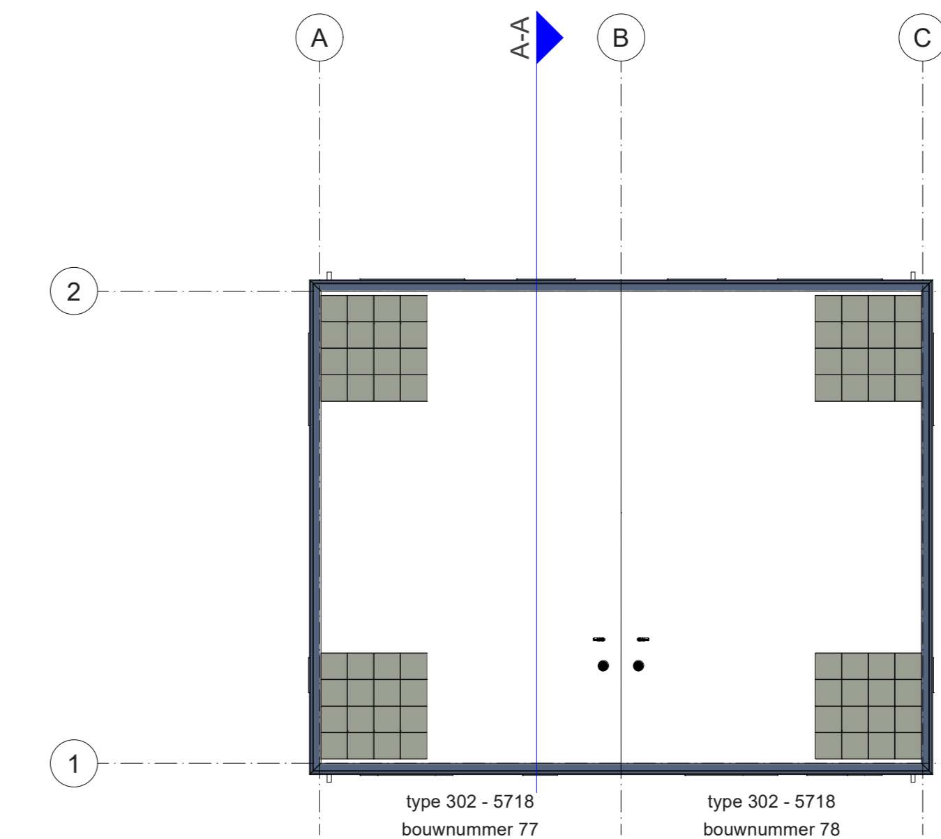
Dak
