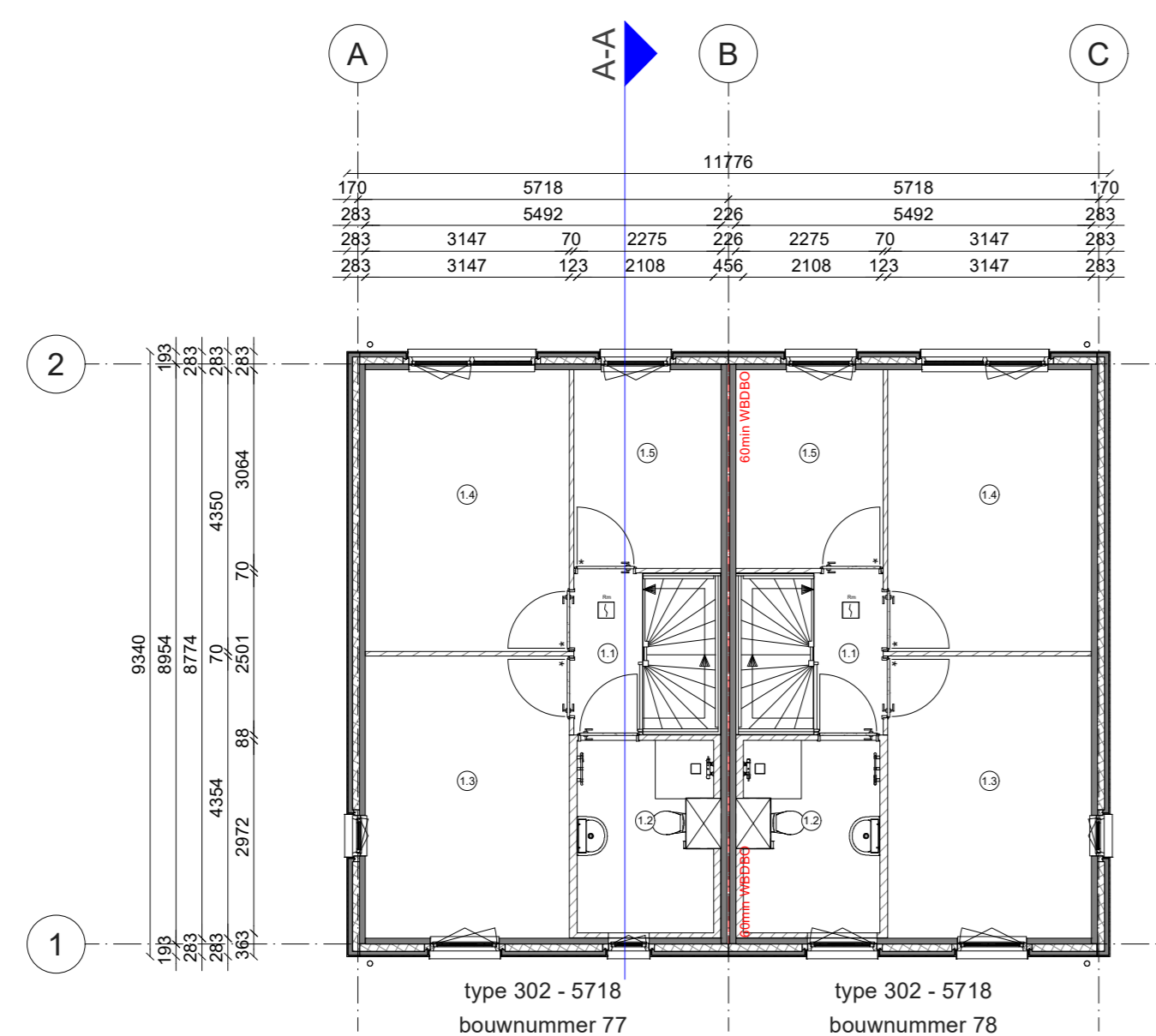
1e Verdieping
