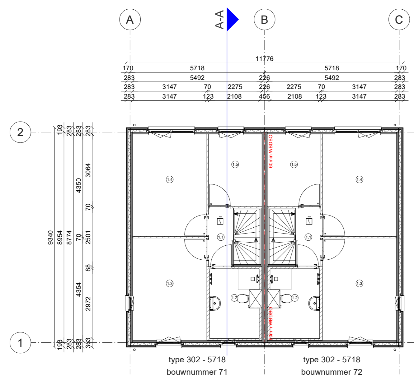
1e Verdieping
