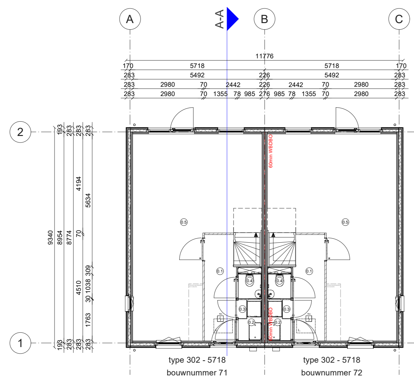
Begane grond
