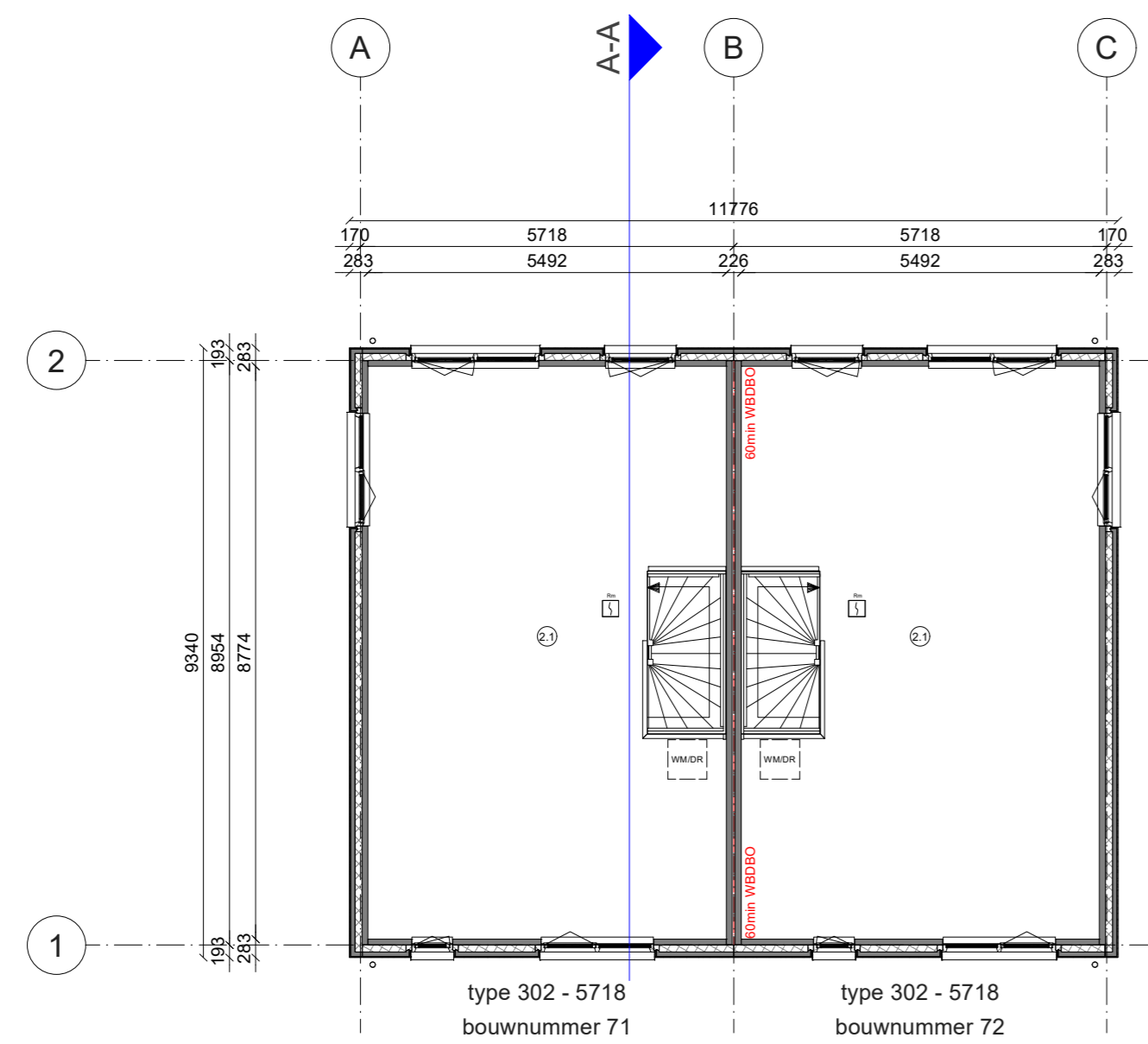
2e Verdieping
