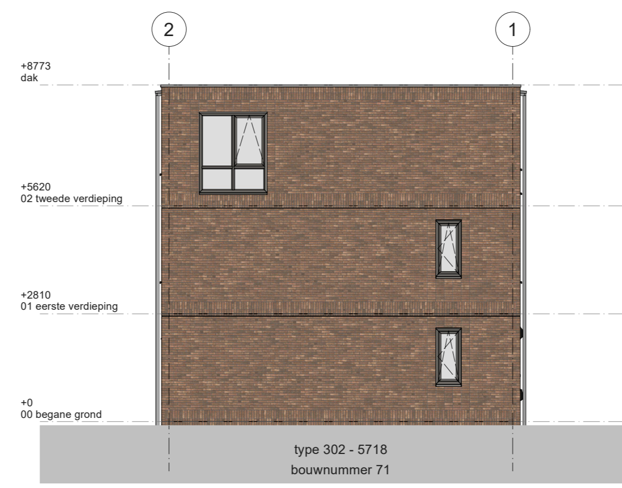
Linkergevel
