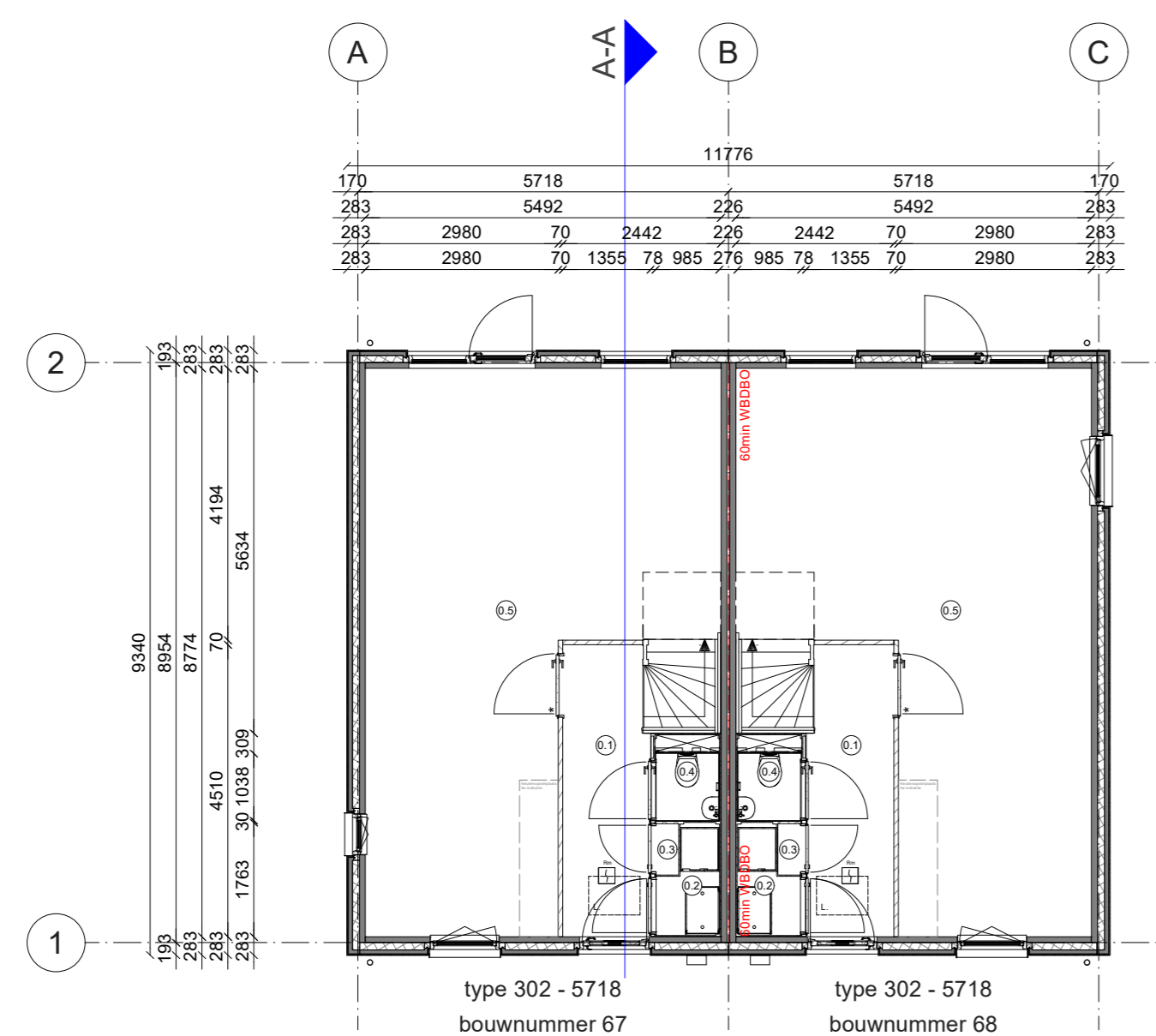
Begane grond
