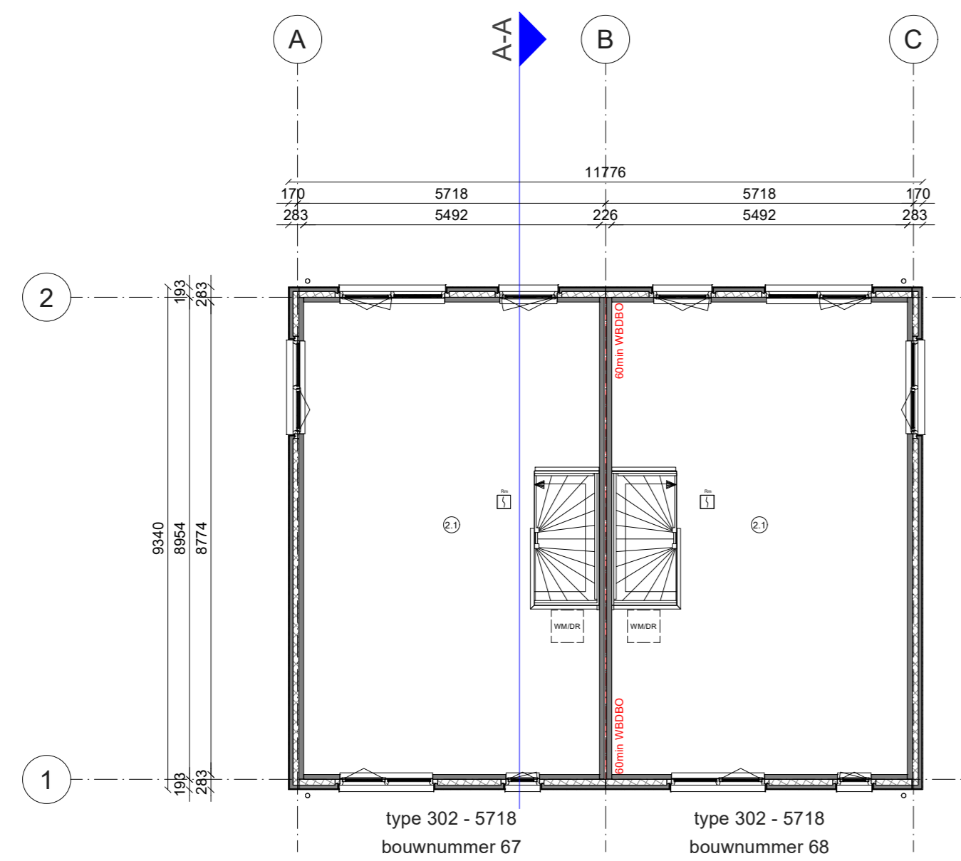
2e Verdieping
