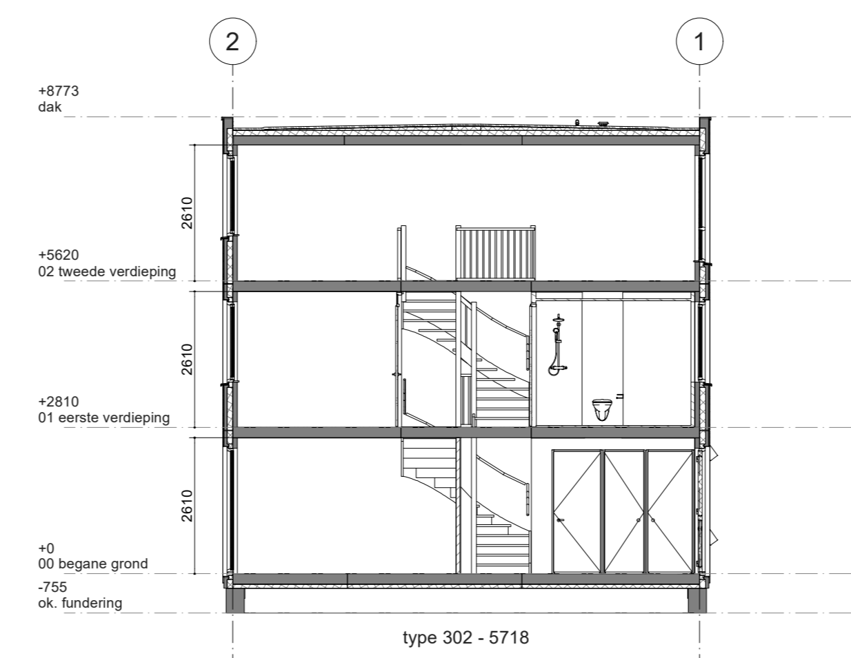
A-A
