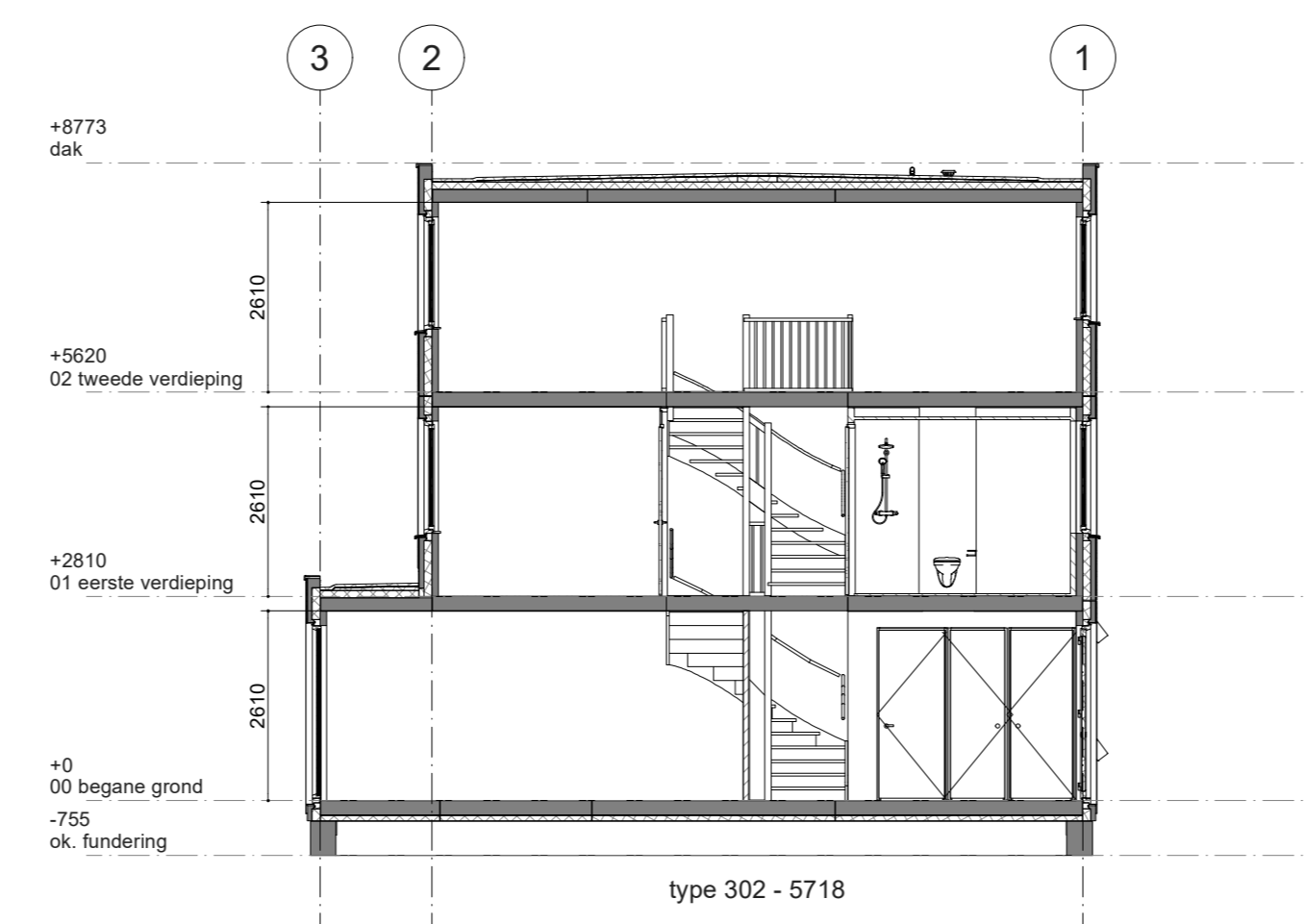
A-A
