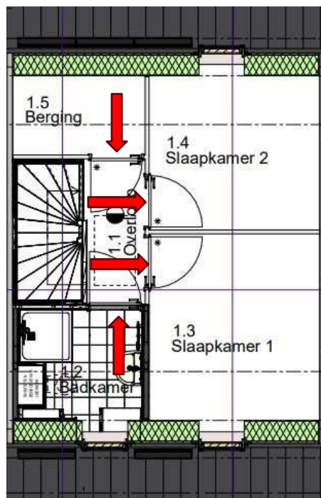
Indeling eerste verdieping met twee slaapkamers en één berging
