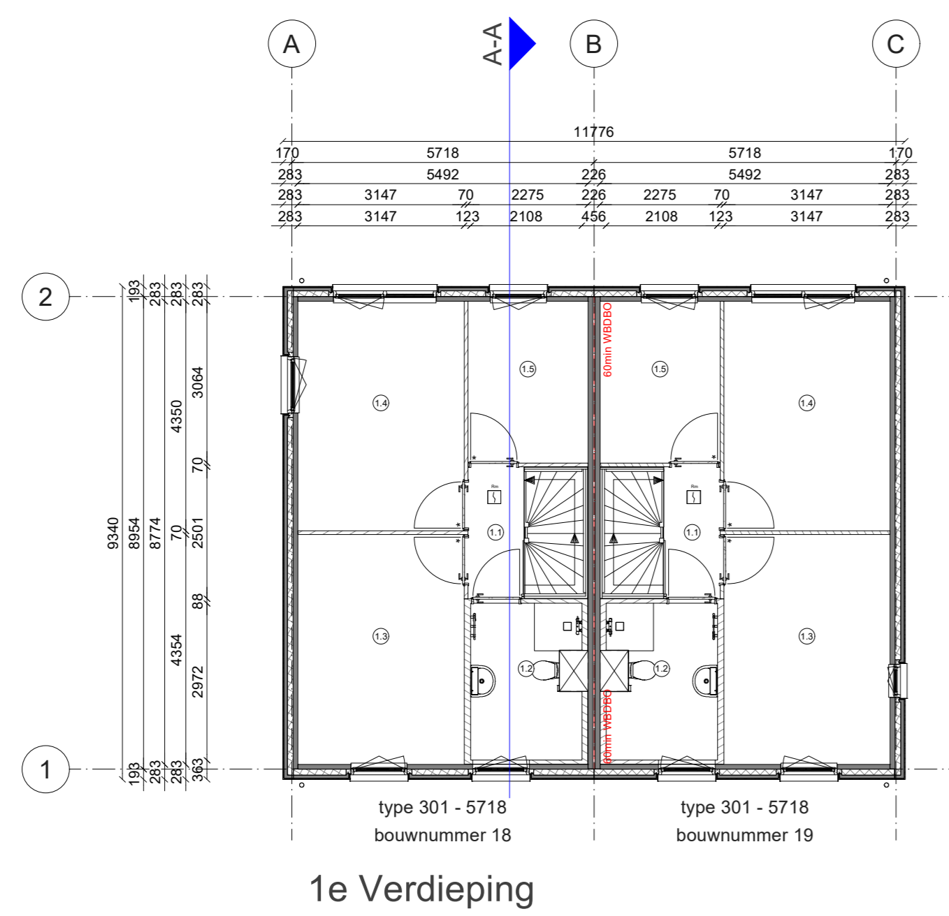
1e Verdieping
