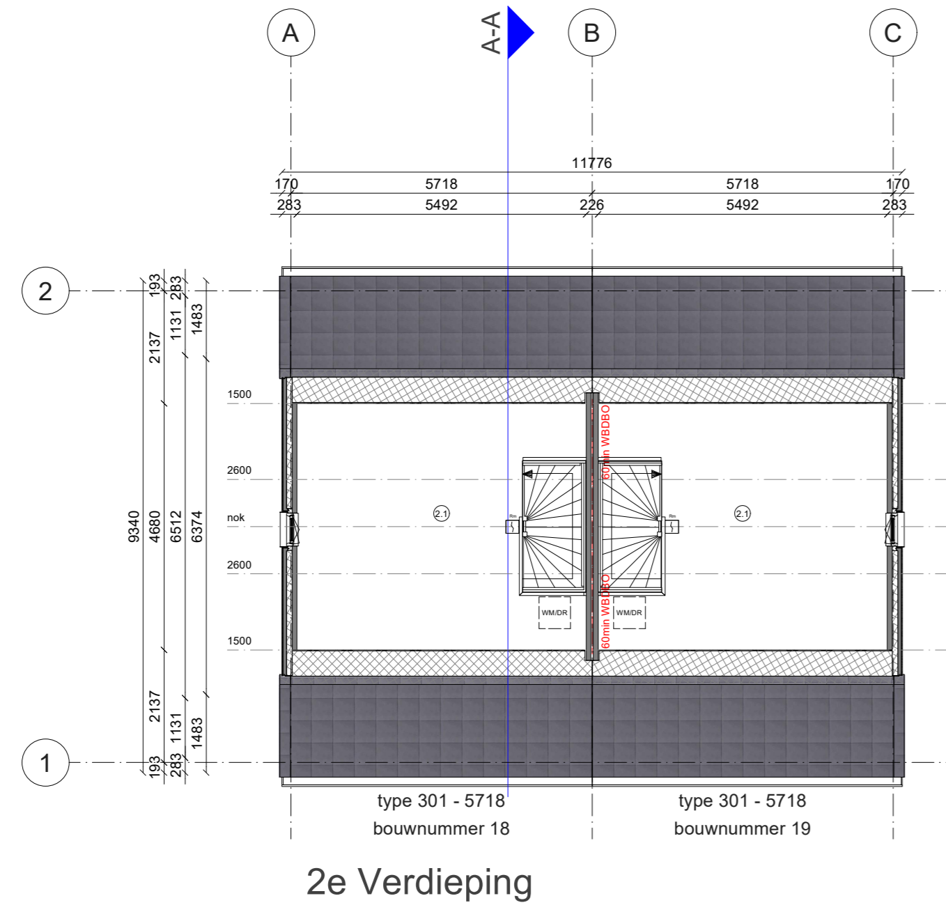
2e Verdieping
