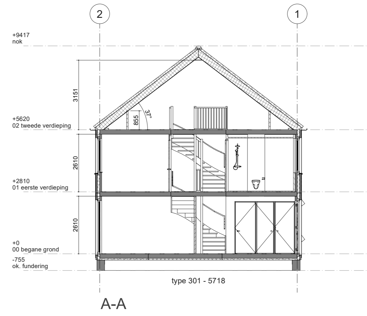
A-A
