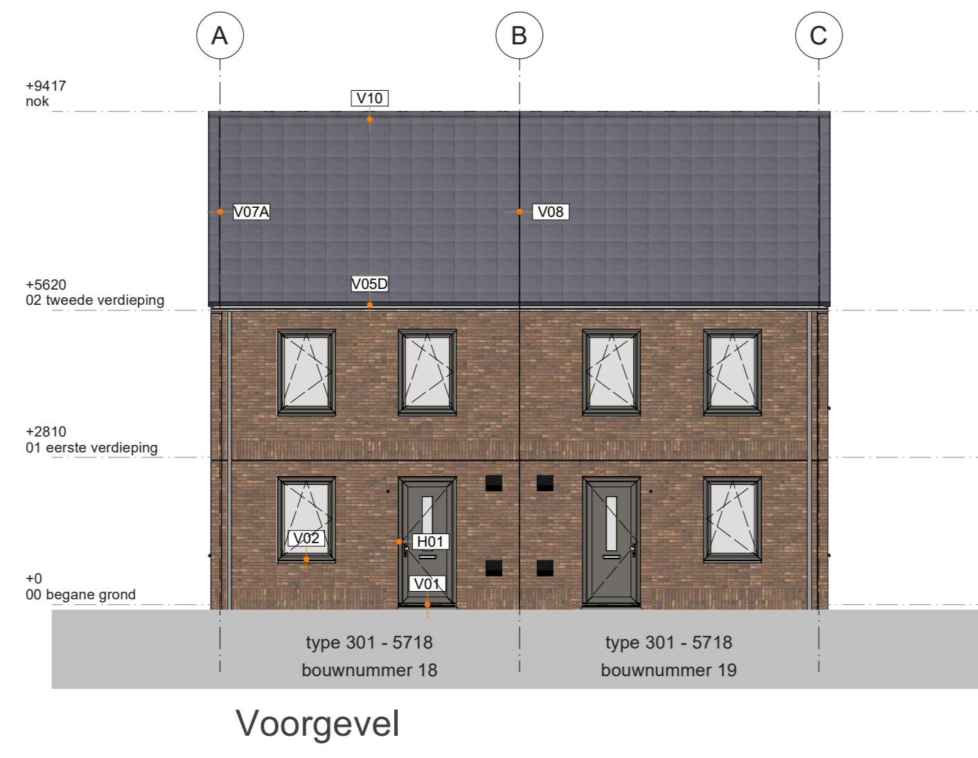
Voorgevel
